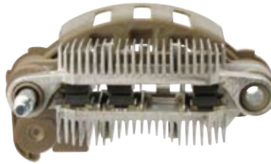
236741 Rectifier
